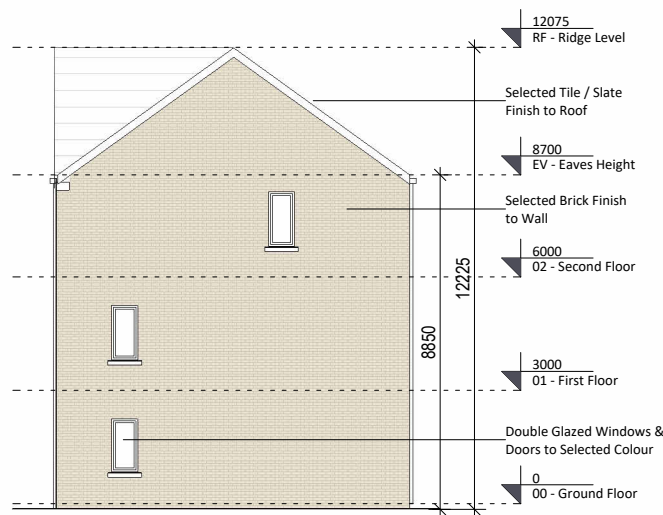
⑥ Right Elevation 1 : 200
