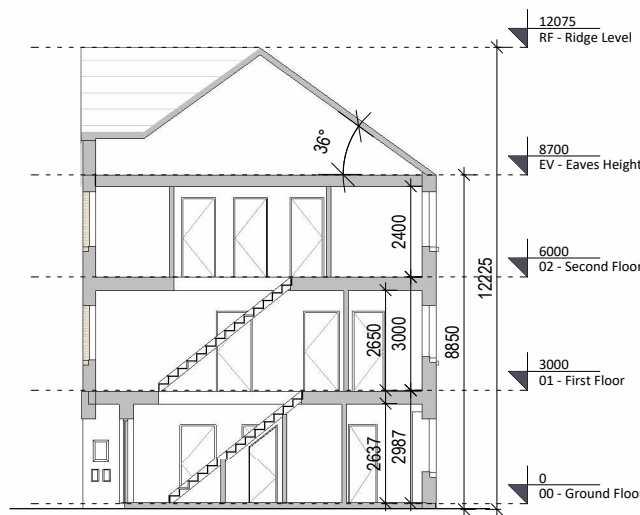
⑦ Section AA 1 : 200
