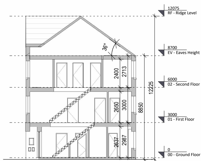
⑥ Section AA 1 : 200
