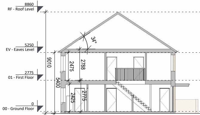
5 Section AA 1 : 200
