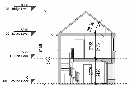
6 Section AA 1 : 200
