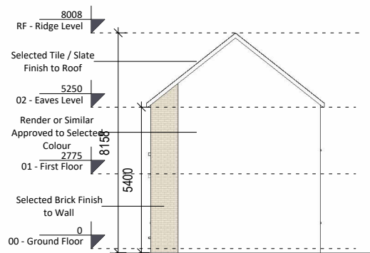
5 Right Elevation 1 : 200
