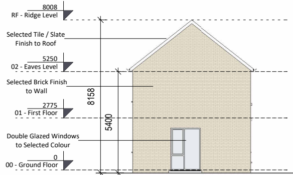
5 Left Elevation 1 : 200
