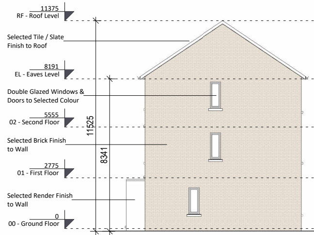
⑥ Right Elevation 1 : 200
