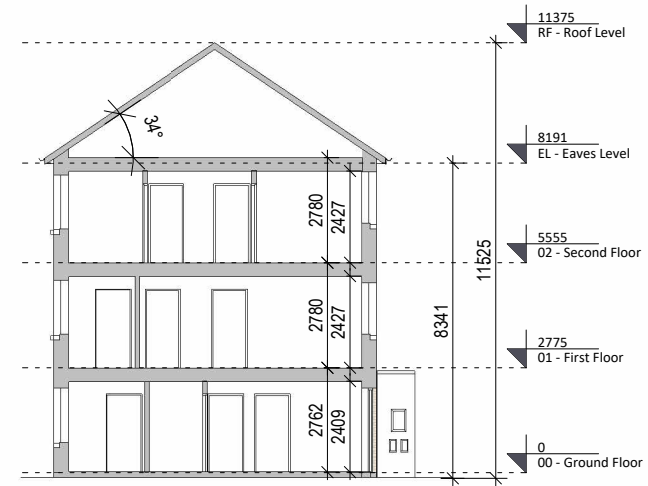
⑦ Section AA 1 : 200
