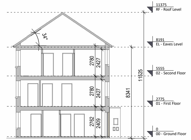
6 Section AA 1 : 200
