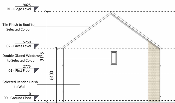
5 Left Elevation 1 : 200
