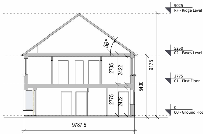
6 Section AA 1 : 200
