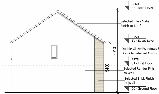
5 Left Elevation 1 : 200
