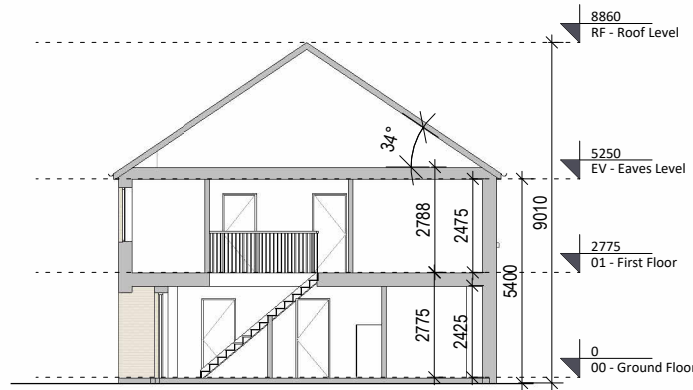
6 Section AA 1 : 200
