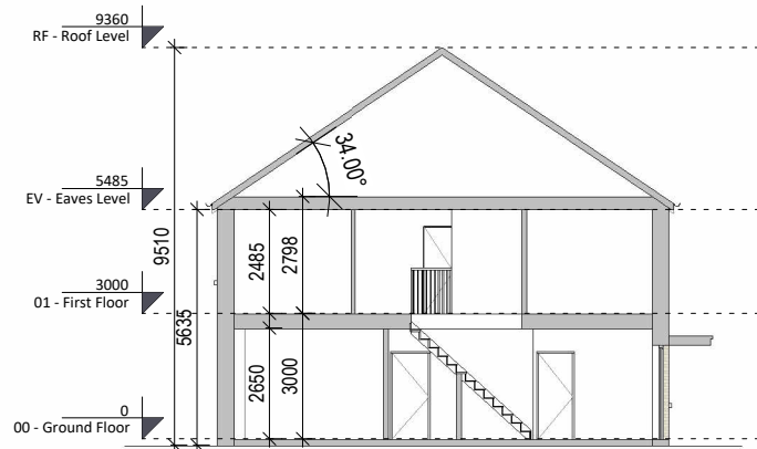
6 Section AA 1 : 200
