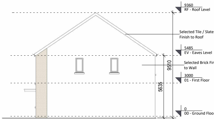
5 Right Elevation 1 : 200
