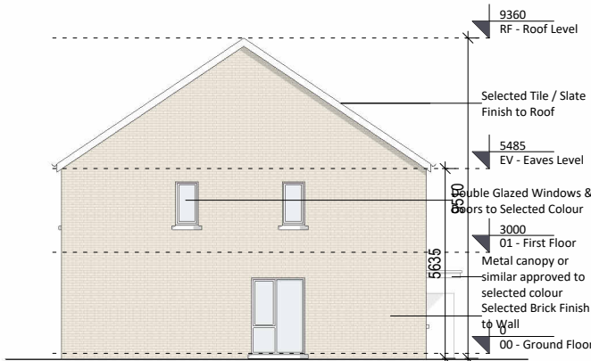
5 Left Elevation 1 : 200
