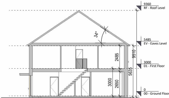
6 Section AA 1 : 200
