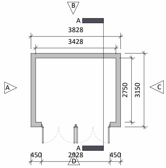
15 Floor Plan 1 : 100
