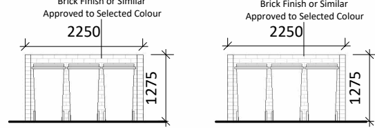
10 Elevation A 1 : 100
