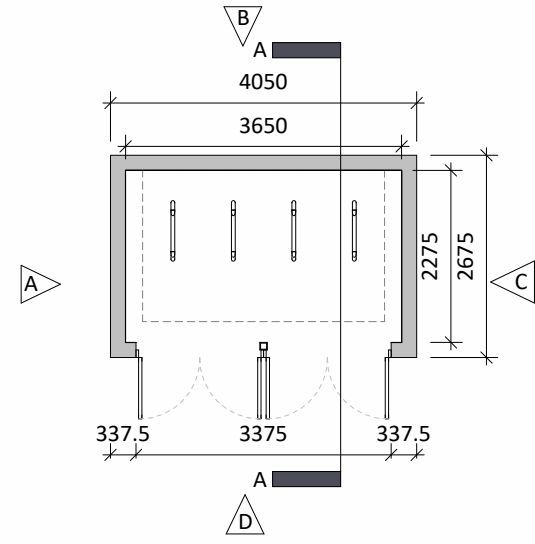
22 Floor Plan 1 : 100
