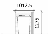
7 Section A-A 1 : 100
