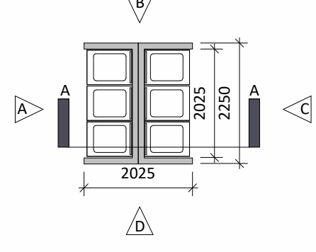
8 Floor Plan 1 : 100
