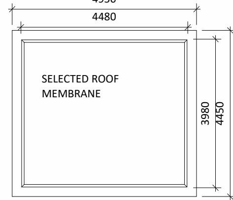
29 Roof Plan 1 : 100
