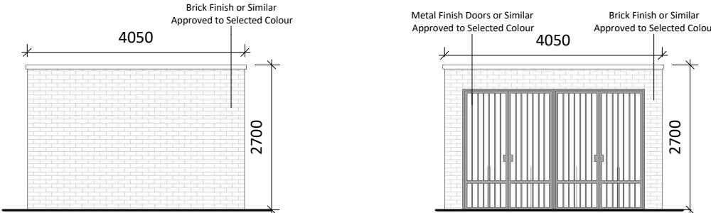
26 Elevation B 1 : 100
