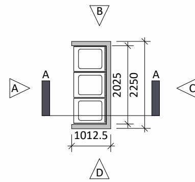
1 Floor Plan 1 : 100
