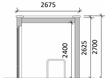
28 Section A-A 1 : 100
