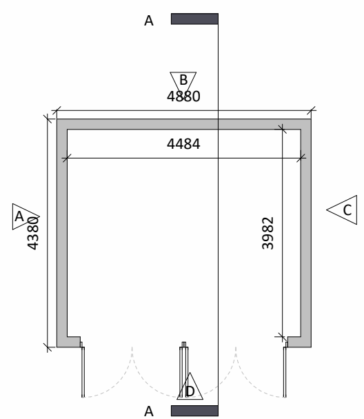
30 Floor Plan 1 : 100
