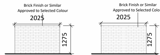
12 Elevation B 1 : 100
