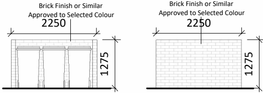
3 Elevation A 1 : 100
