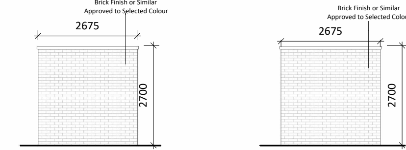
24 Elevation A 1 : 100
