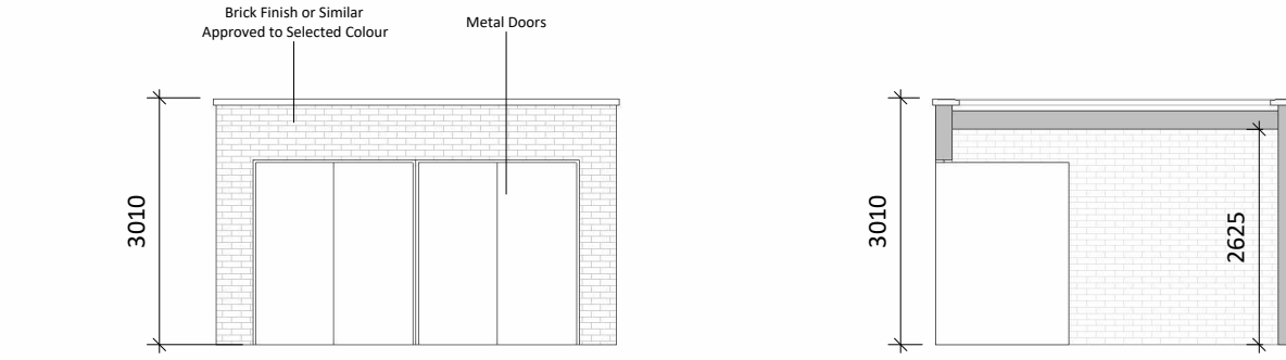
34 Elevation D 1 : 100
