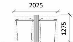
14 Section A-A 1 : 100
