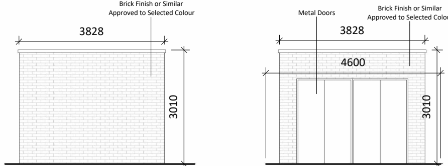
19 Elevation B 1 : 100
